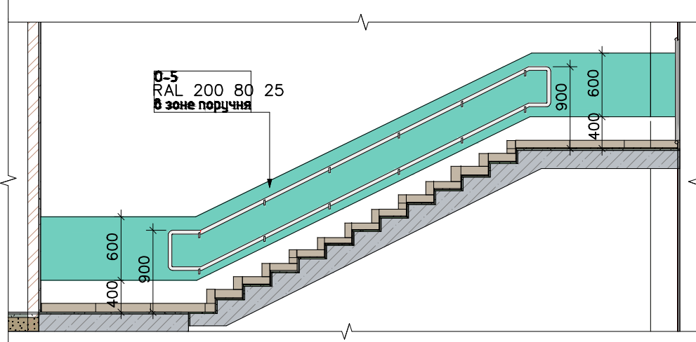
Схема окраски стен в зоне поручня ЛК
